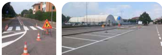
Segnaletica orizzontale
